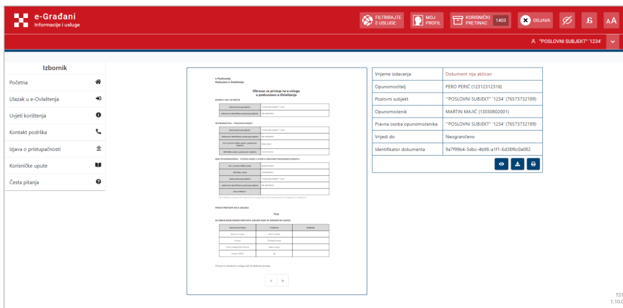
Slika 71. Ispis dokumenta
