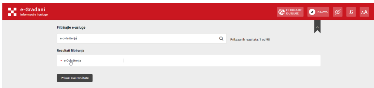
Slika 1. Pristup usluzi
