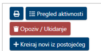
Slika 70. Dodatne opcije
