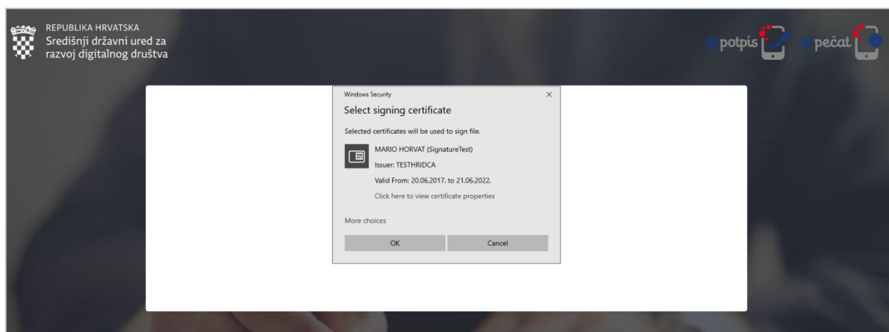
Slika 83. Odabir certifikata
